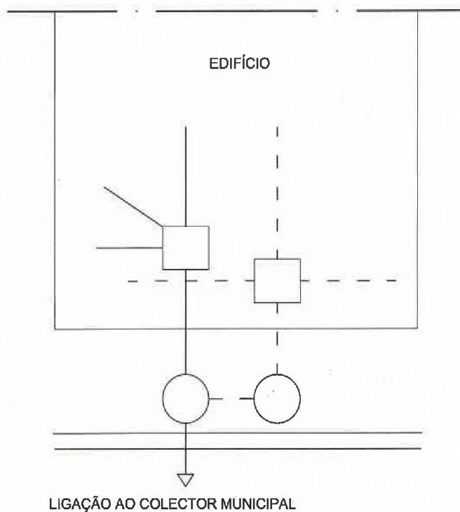
REDE UNITÁRIA
