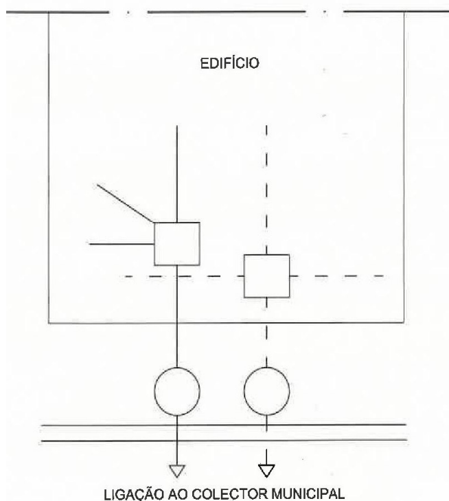
REDE SEPARATIVA
